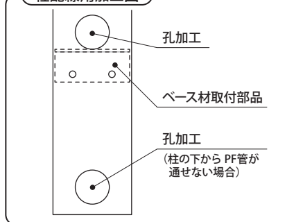
柱配線用加工図
