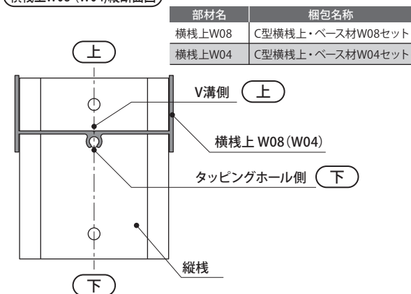
横棧上W08 (W04) 縦断面図
