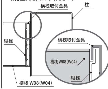
横棧W08 (W04)・横棧取付金具納まり図
