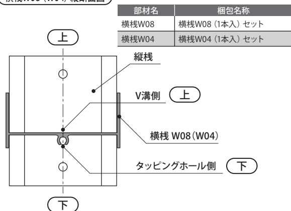
横棧W08 (W04) 縦断面図
